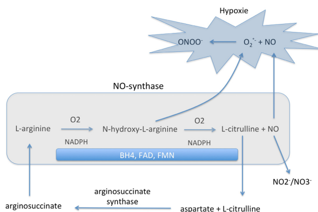
Fig. 1 Représentation schématique du métabolisme du monoxyde d'azote (NO) et de ses principaux dérivés. La production de NO et de citrulline est assurée par des NO synthases à partir de L-arginine et nécessite plusieurs cofacteurs : nicotinamide adénine dinucléotide phosphate (NADPH), tétrahydrobioptérine (BH4), flavine adénine dinucléotide (FAD), flavine mononucléotide (FMN). Dans certaines conditions, la citrulline peut être recyclée en L-arginine par l'arginosuccinate synthase (cycle arginine-citrulline). Le NO peut donner naissance au peroxy-nitrite ( \text{ONOO}^- ) par conjugaison avec l'anion superoxyde ( \text{O}_2^- ). Les nitrates ( \text{NO}_2^- ) et nitrites ( \text{NO}_3^- ) sont d'autres métabolites actifs du NO.
